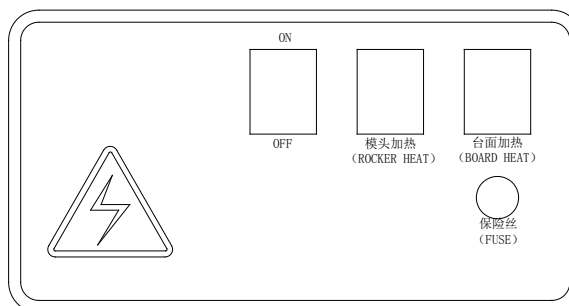
Рис. 2 Панель управления гладильного стола.
