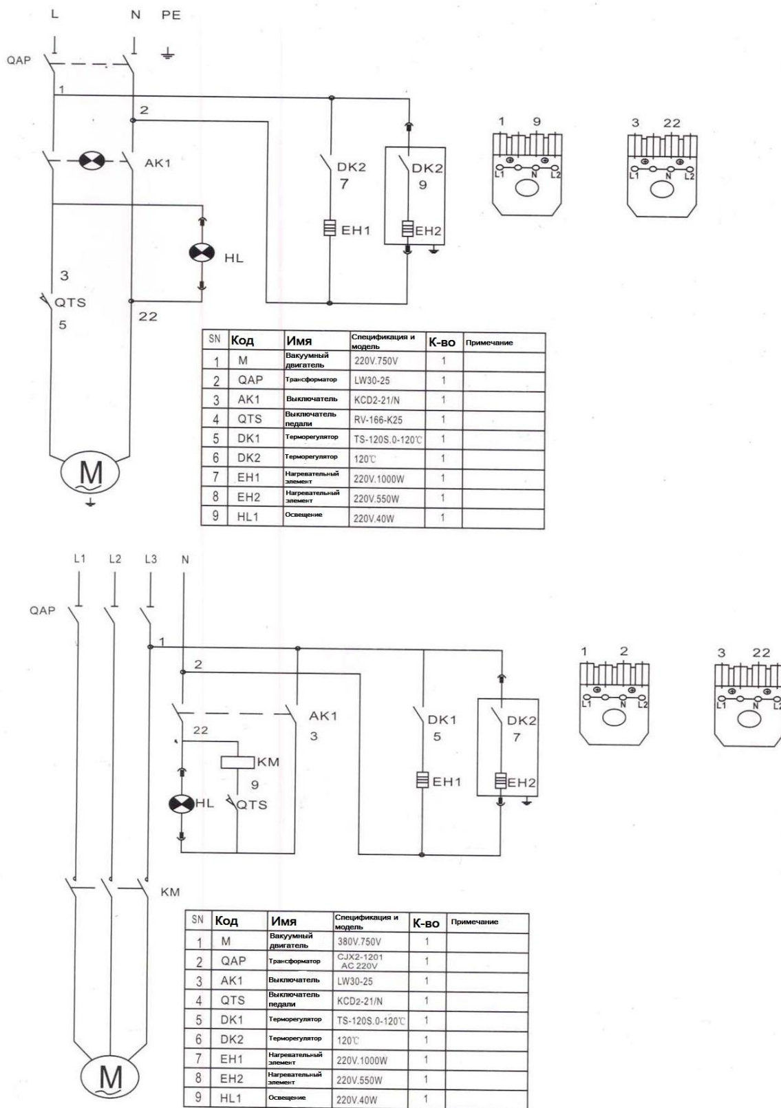
Рис. 4. Электрическая схема гладильного стола JT-TDZ-QII-QIV
