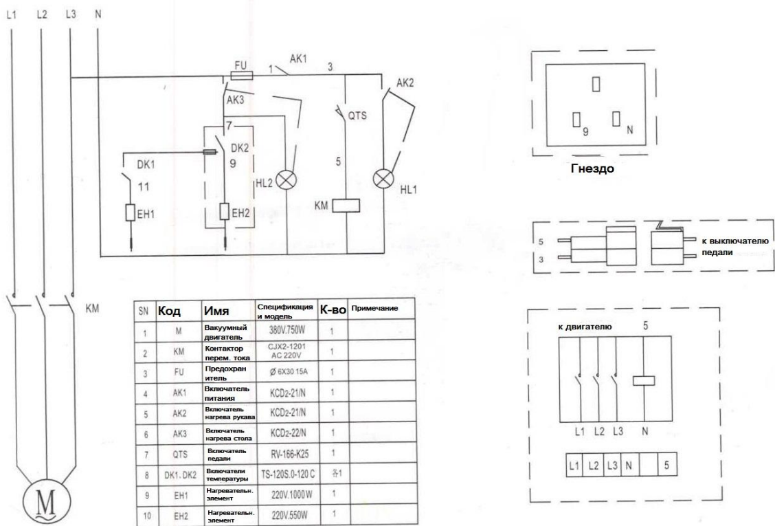
Рис. 3. Электрическая схема гладильного стола JT-TDZ-Q1
